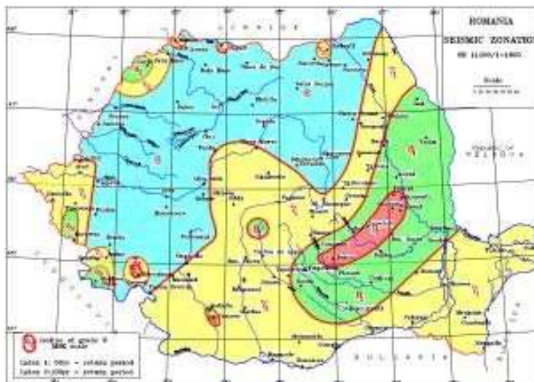
Figura 6 – Zonarea seismică SR 1100-1:93
