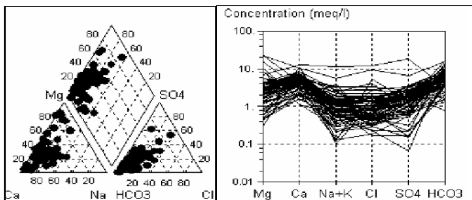
Diagramele Piper și Schoeller efectuate pe baza analizelor chimice ale forajelor existente în zona corpului de apă (Corpul ROJ105)
