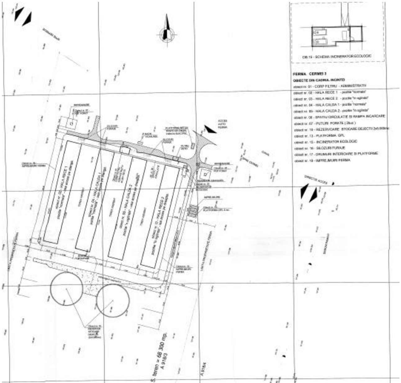
Figura 1: Plan de amplasament cu traseele rețelilor de canalizare
